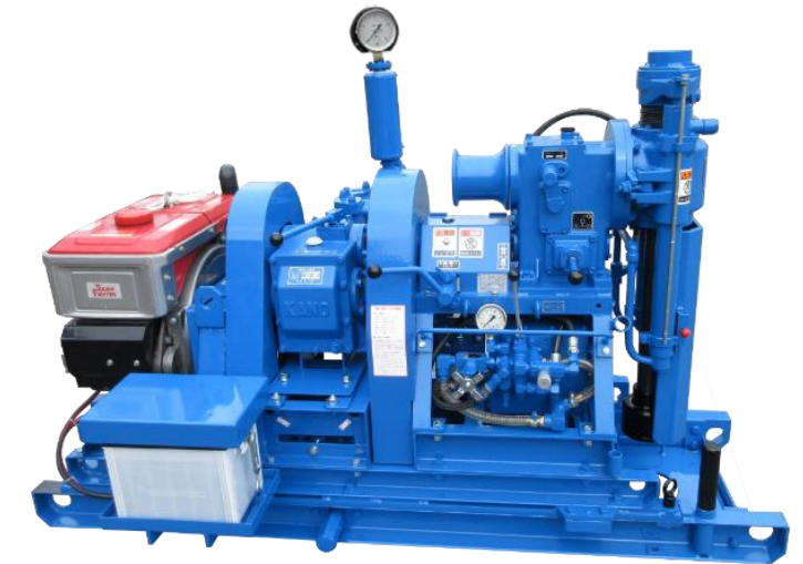
☆KR-SH-2V5-S4-M（特注） スピンドルストローク400mm V5-P 手動式スライドベース付（特注）
