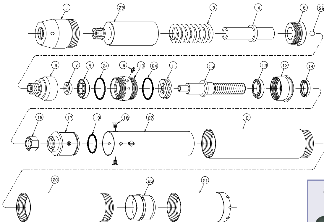
デニソンサンプラー改造型分解図
